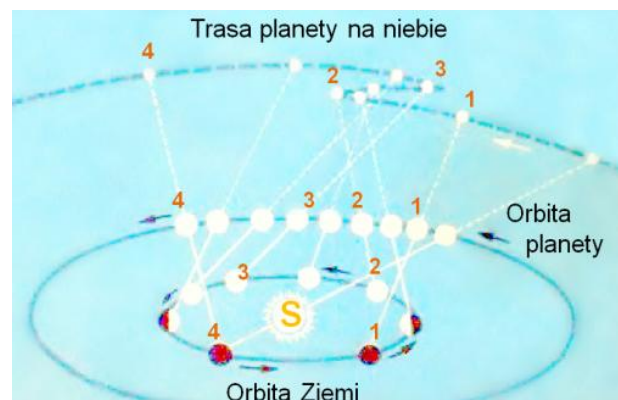
Ryc. 2. Orbity Ziemi i planety zewnętrznej wokół Słońca. Planeta zewnętrzna jest w większej
