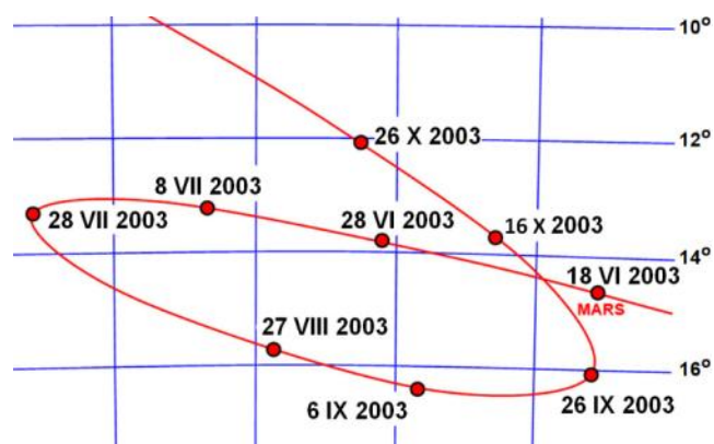
Ryc. 1. Droga Marsa na sferze niebieskiej.
