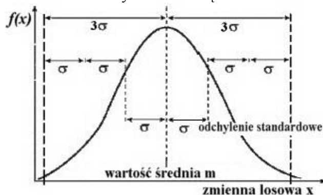
Wykres funkcji Gaussa.
